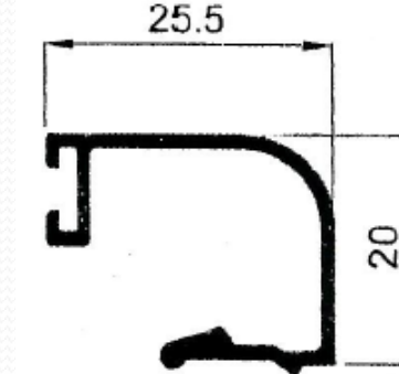
8214 – Junquillo curvo 25,5 mm.
