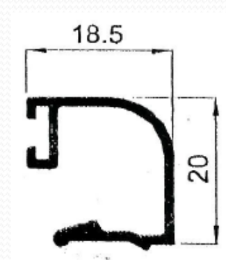
8213 – Junquillo curvo 18,5 mm.
