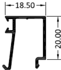
2108 – Junquillo recto 18,5 mm.
