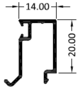
5609 – Junquillo recto 14 mm.
