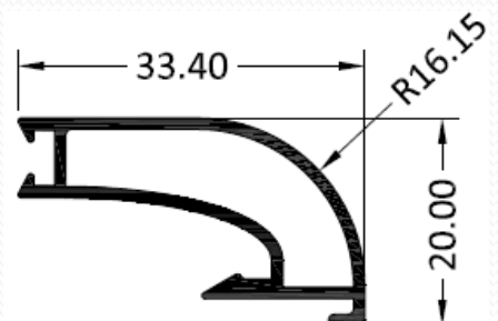
3856 – Junquillo curvo 33,4 mm.
