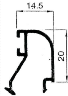
8276 – Junquillo curvo clip 14,5 mm.
