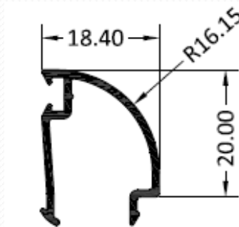
3821 – Junquillo curvo clip 18,4 mm.
