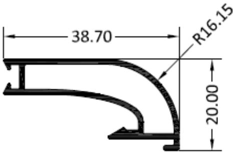
3871 – Junquillo curvo 38,7 mm.
