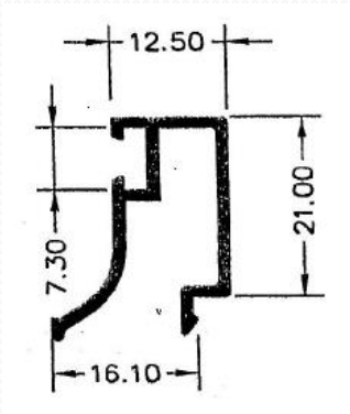
5812 – Junquillo recto 28,2 mm.
