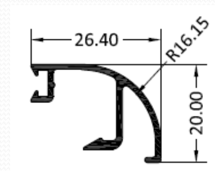
3833 – Junquillo curvo 26,4 mm.
