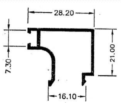
5812 – Junquillo recto 28,2 mm.
