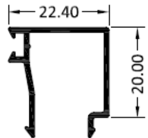
3826 – Junquillo recto 22,4 mm.
