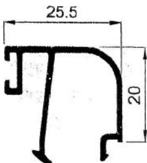
8278 – Junquillo curvo clip 25,5 mm.
