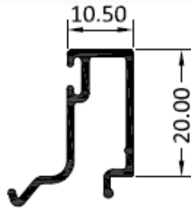
5921 – Junquillo recto 10,5 mm.
