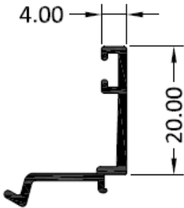
5343 – Junquillo recto 4 mm.
