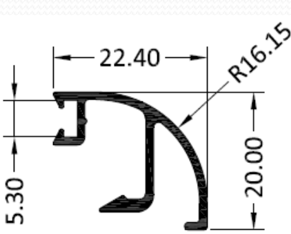
3834 – Junquillo curvo 22,4 mm.
