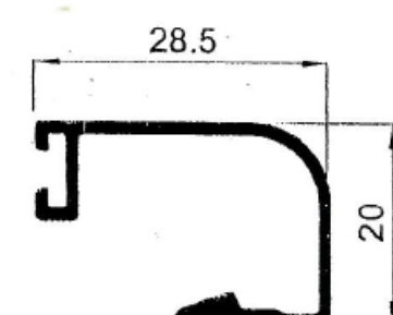
8452 – Junquillo curvo 28,5 mm.
