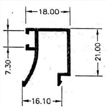
9022 – Junquillo recto 18 mm.
