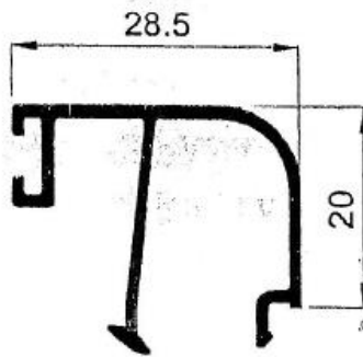
8257 – Junquillo curvo clip 28,5 mm.
