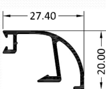
3857 – Junquillo curvo 27,4 mm.
