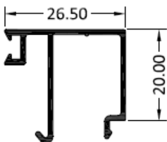
2109 – Junquillo recto 26,5 mm.
