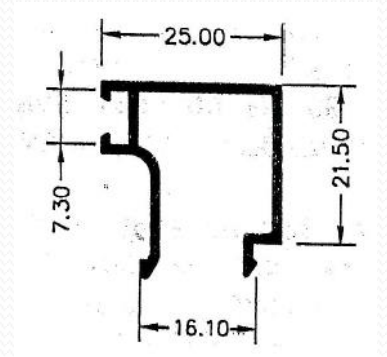
9021 – Junquillo recto 25 mm.
