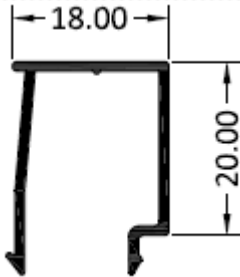
3832 – Junquillo recto 18 mm.
