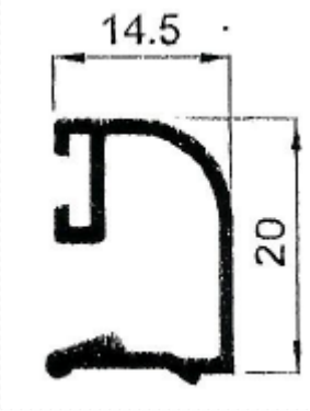
8277 – Junquillo curvo 14,5 mm.
