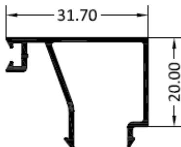
2777 – Junquillo recto 31,7 mm.
