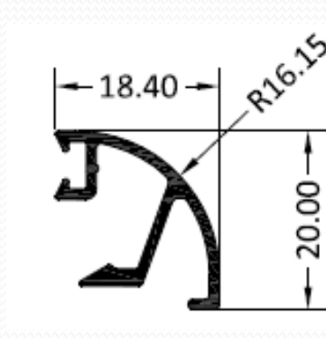
3822 – Junquillo curvo 18,4 mm.
