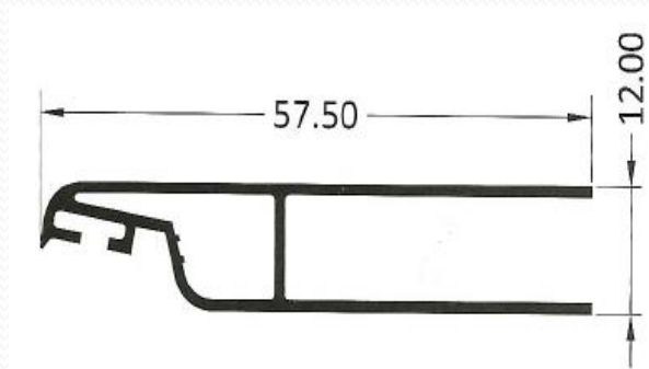
4411 – Lama fija
