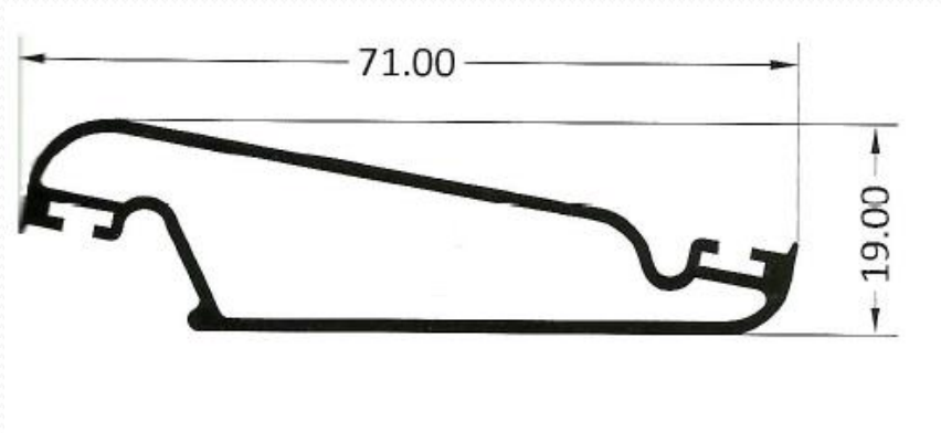
4412 – Lama móvil
