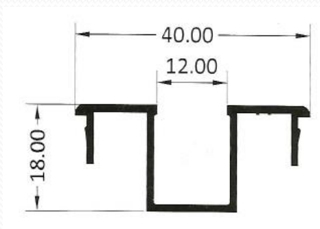
3658 – Perfil base
