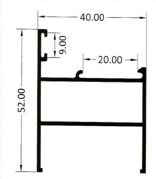
3650 – Hoja mallorquina
