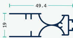
02 Guía de Deslizamiento
