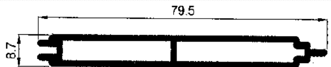
6644 – Lama Postigo 79,5 mm.
