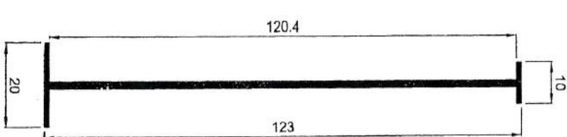
515 – Unión de 120 mm.
