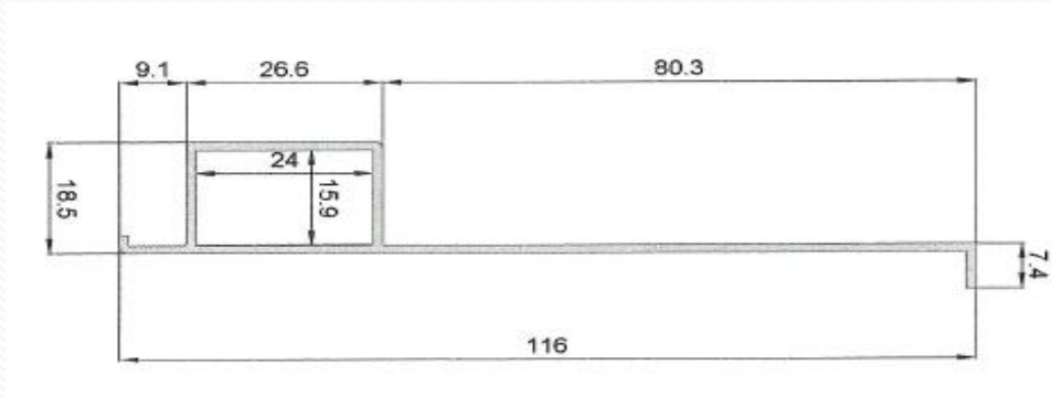
00342P – Premarco de 120 mm. ala invertida
