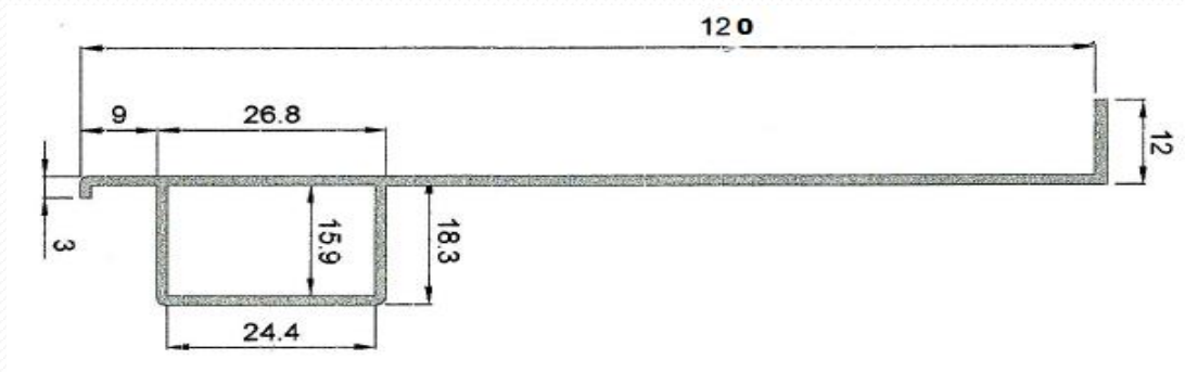
4218 – Premarco de 120 mm.
