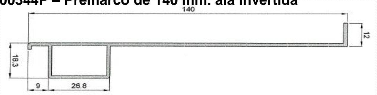
00344P – Premarco de 140 mm. ala invertida
