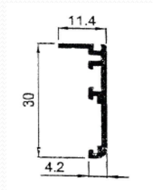
4378 – Solape clip de 30 mm. E4089 – Solape guía de 30 mm.
