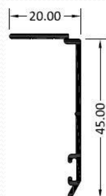
4376 – Solape clip de 45 mm. 4377 – Solape guía de 45 mm.
