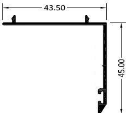
4376 – Solape clip de 45 mm. 4377 – Solape guía de 45 mm.
