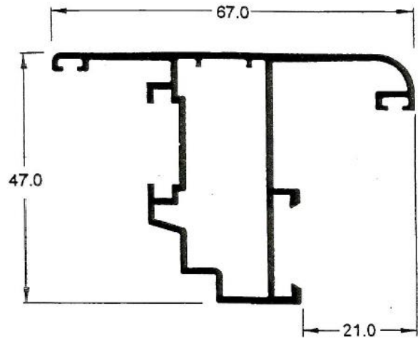
5206 – Hoja de ventana de apertura externa
